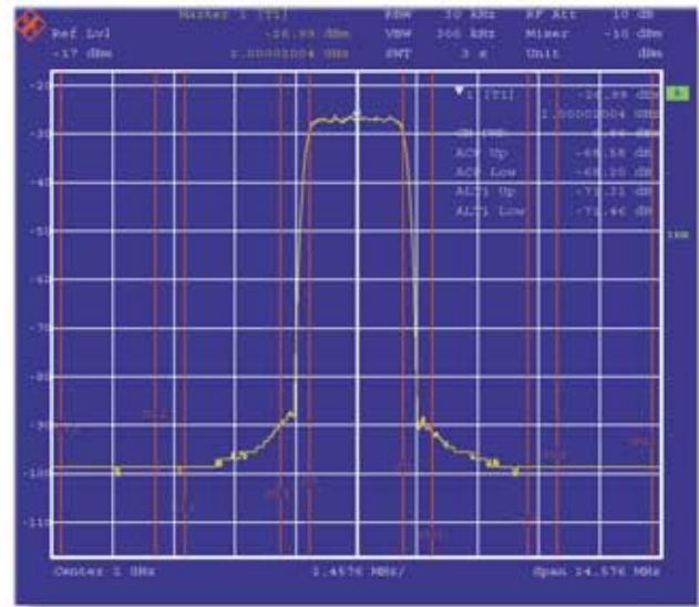
WCDMA spectrum
